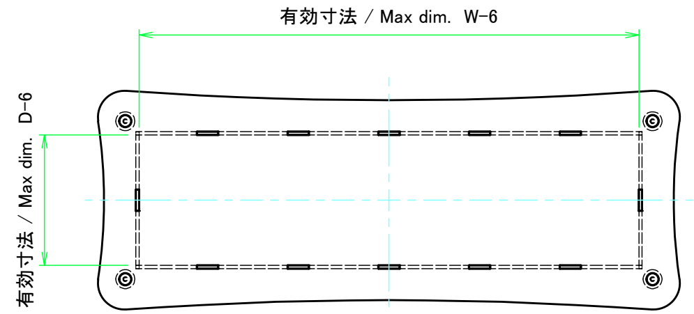
下カバー / Bottom cover
