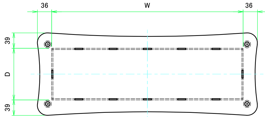
上カバー / Top cover
